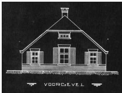
fig. 9a Bouwtekening van het huis van Nijenhuis
